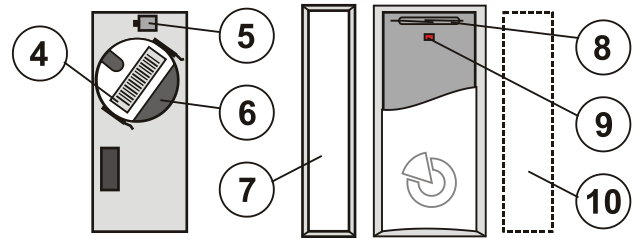
Afbeelding 3: 4 - productiecode 5 – sabotagecontact; 6 – batterij; 7 – permanente magneet; 8 – magnetische sensor; 9 – rode activeringsindicator; 10 – alternatieve plaats voor de permanente magneet
