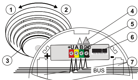
Afb. 6: 1 – het openen van het detectordekseel; 2 – het sluiten van het detectordekseel; 3 – signalering van de optische status; 4 – de pijl, die aangeeft, dat de detector geplaatst dient te worden; 5 – busterminiaal; 6 – productiecode 7 – batterijhouders
